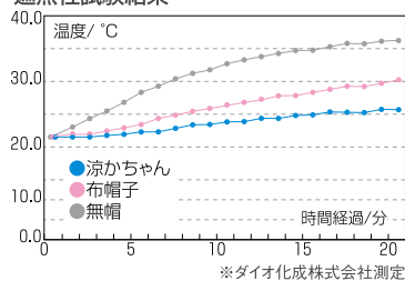
遮熱性試験結果
